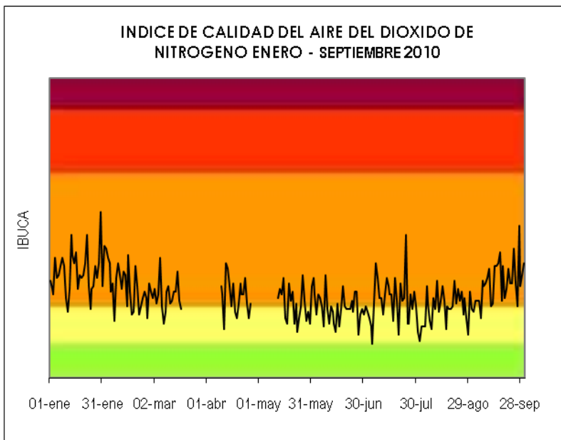
Fig 5. Comportamiento NO 2 entre enero – septiembre 2010
