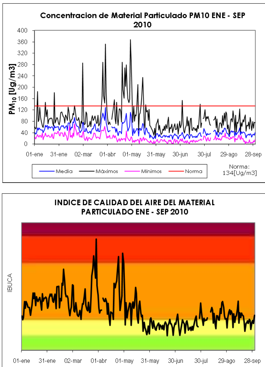
Fig 3. Comportamiento PM10 entre enero – septiembre 2010
