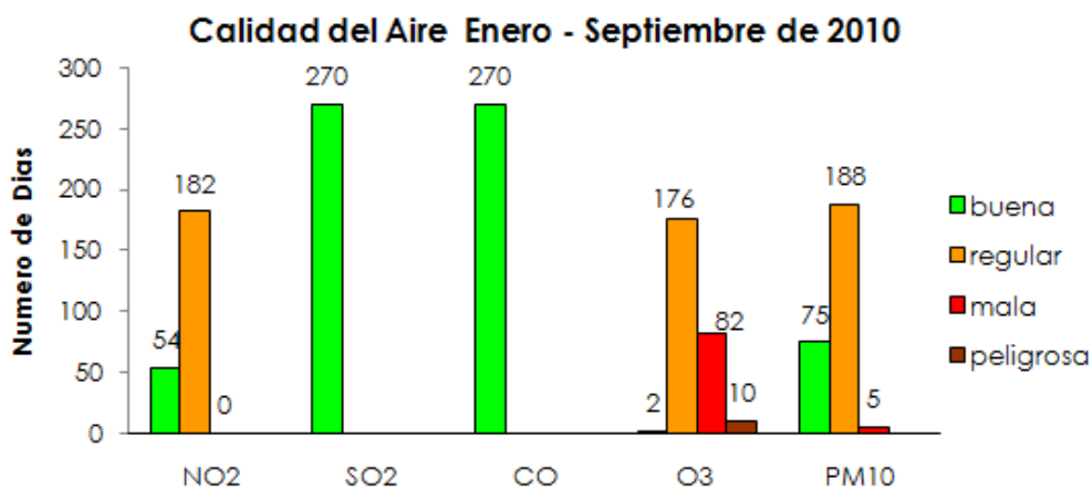
Fig 2. Grafica IBUCA en el AMB entre enero – septiembre 2010
