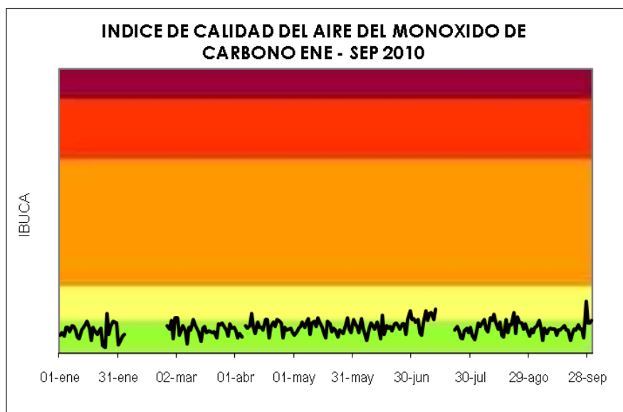
Fig 6. Comportamiento CO entre enero – septiembre 2010
