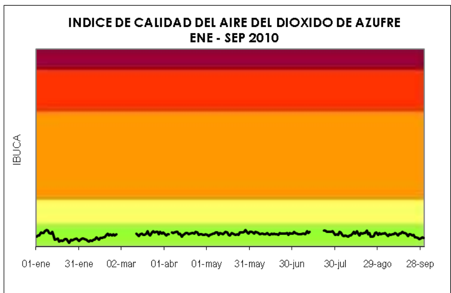
Fig 7. Comportamiento SO 2 entre enero – septiembre 2010
