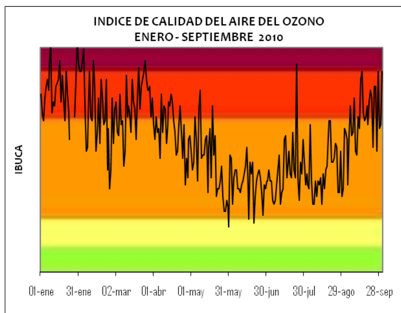
Fig 4. Comportamiento O 3 entre enero – septiembre 2010
