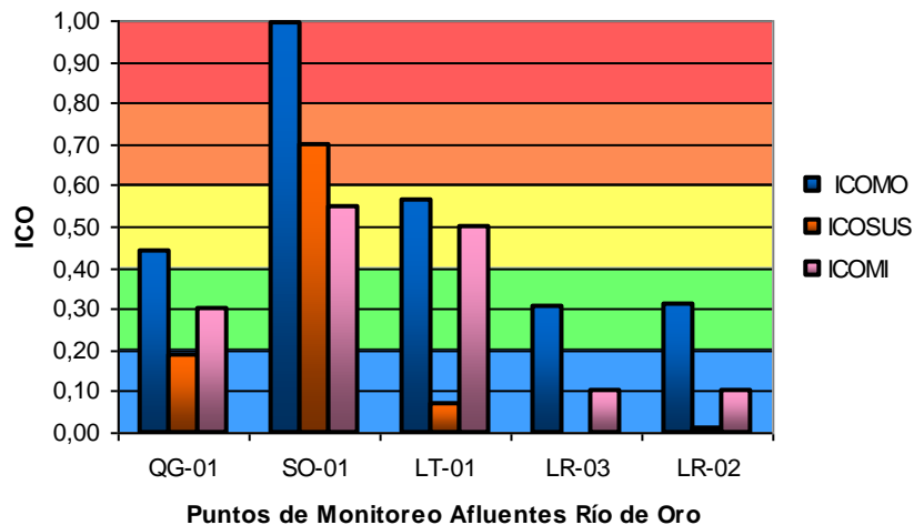
Gráfica 12. Promedio semestral Índices de Contaminación del Agua - Afluentes Mcpios Piedecuesta y Girón
