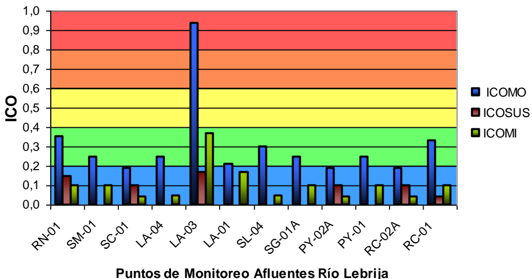
Gráfica 24. Promedio Índices de Contaminación del Agua – Afluentes Río Lebrija
