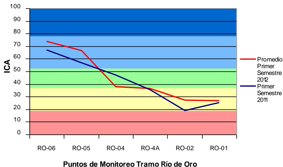
Gráfica 9. Promedio Semestral Índice de Calidad del Agua - Río de Oro
