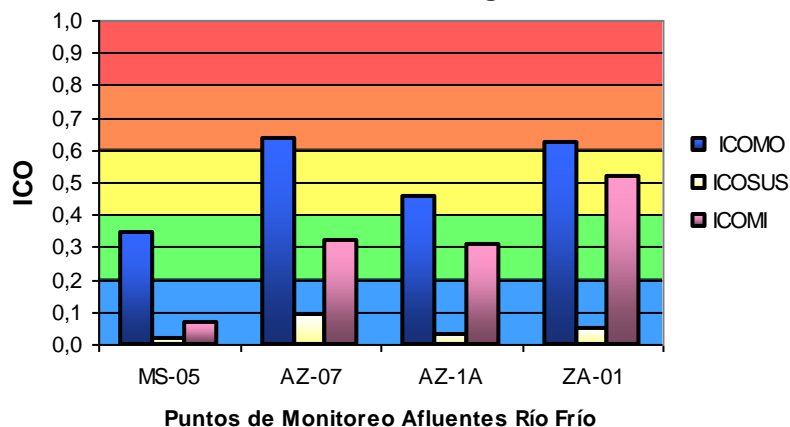
Gráfica 16. Promedio Índices de Contaminación del Agua Semestral 2012- Afluentes Río Frío
