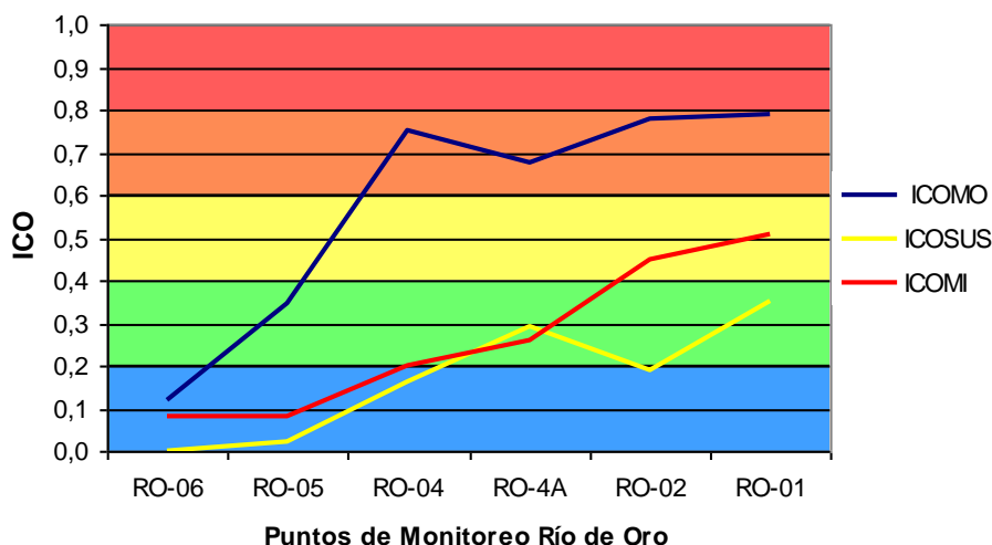
Gráfica 10. Promedio semestral Índices de Contaminación del Agua - Río de Oro
