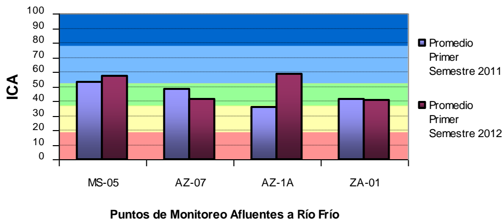
Gráfica 15. Promedio semestral Índice de Calidad del Agua – Afluentes Río Frío
