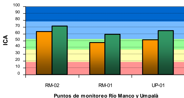
Gráfica 25. Promedio semestral Índice de Calidad del Agua – Ríos Manco y Umpalá
