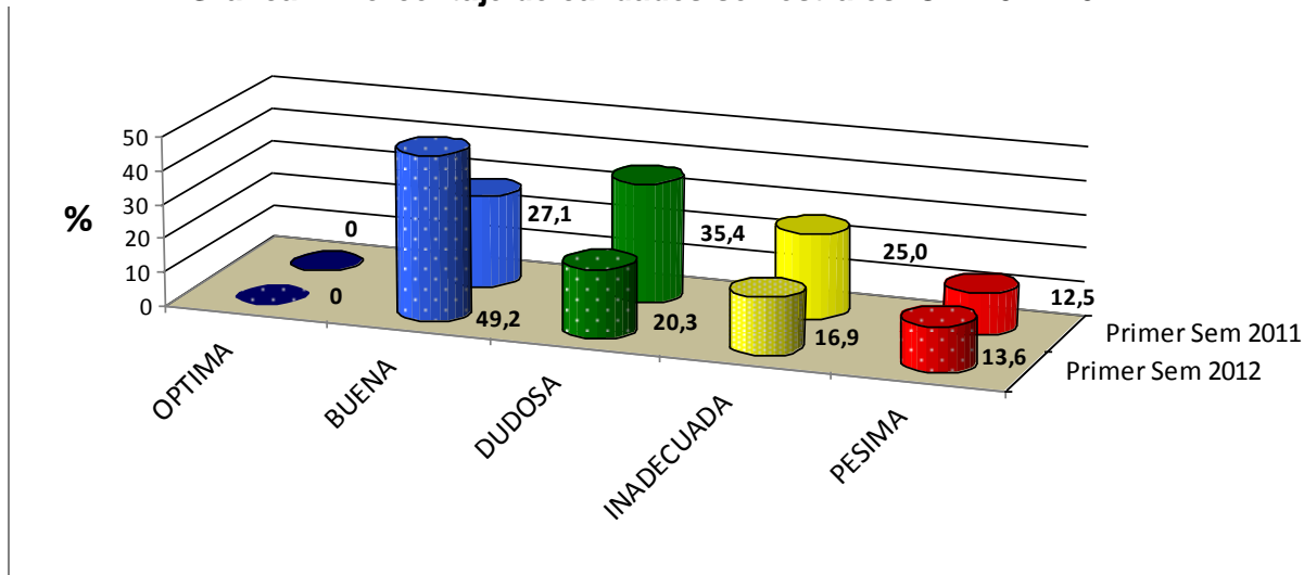
Gráfica 2. Porcentaje de calidades semestrales ICA 2011-2012
