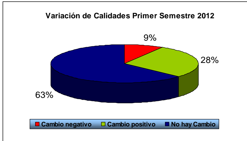
Gráfica 1. Variabilidad en la calidad del agua Primer Semestre 2012
