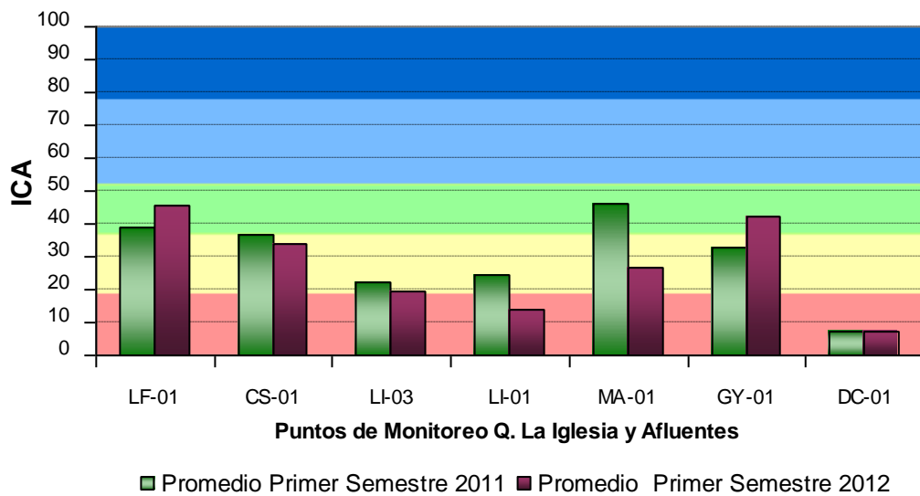
Gráfica 18. Promedio Índices de Contaminación del Agua - Qda La Iglesia y sus afluentes
