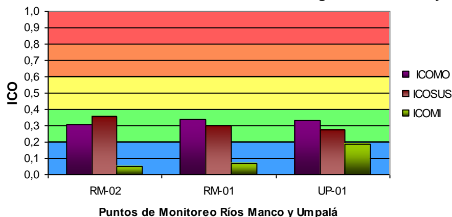
Gráfica 26. Promedio Índices de Contaminación del Agua - Ríos Manco y Umpalá
