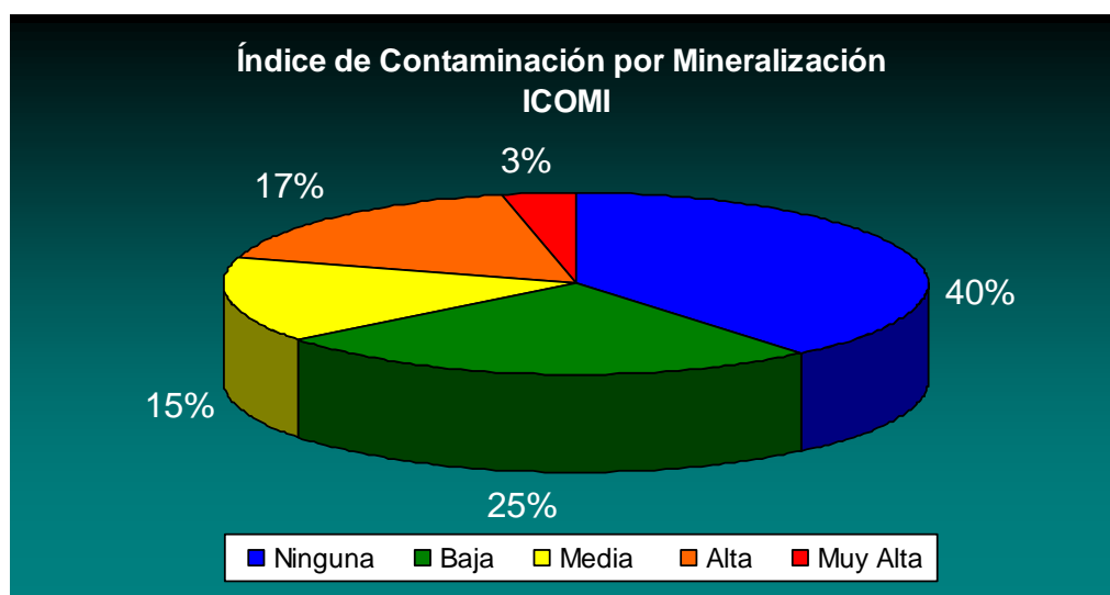
Gráfica 6. Promedio Índice de Contaminación por Mineralización
