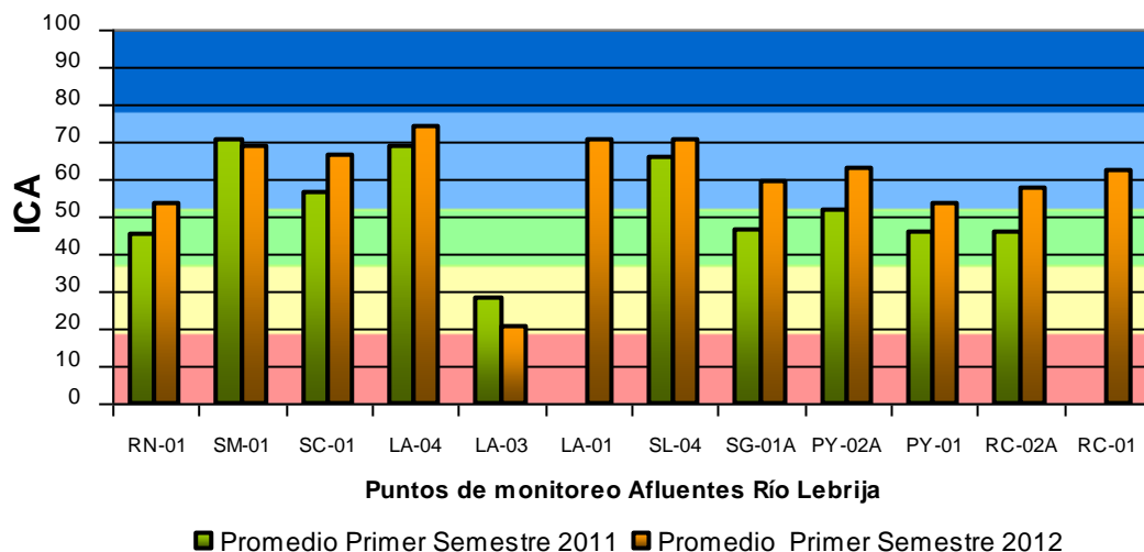
Gráfica 24. Promedio Índices de Contaminación del Agua – Afluentes Río Lebrija
