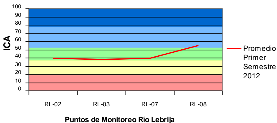
Gráfica 21. Promedio Semestral Índice de Calidad del Agua – Río Lebrija
