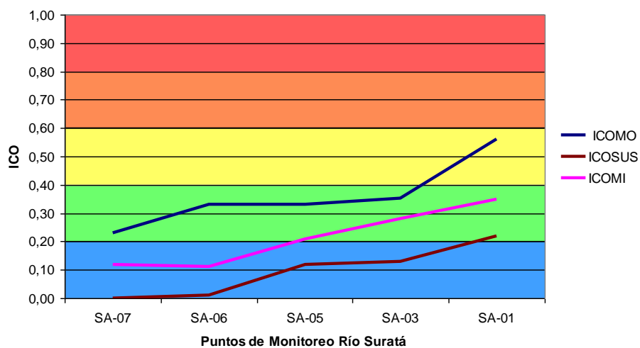
Gráfica 8. Promedio Índices de Contaminación del Agua - Río Suratá
