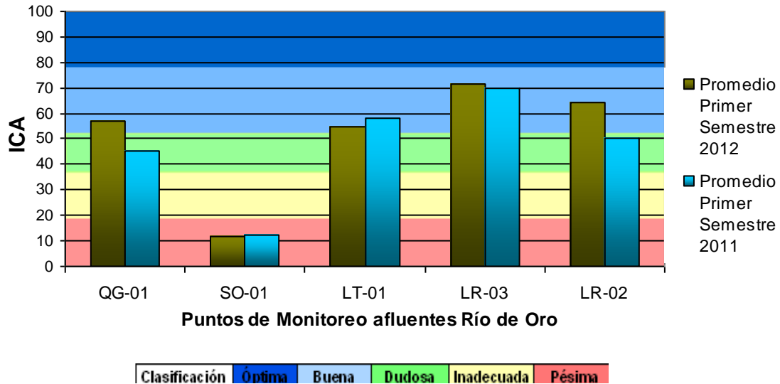
Gráfica 11. Promedio Semestral Índice de Calidad del Agua - Afluentes Mcpios Piedecuesta y Girón
