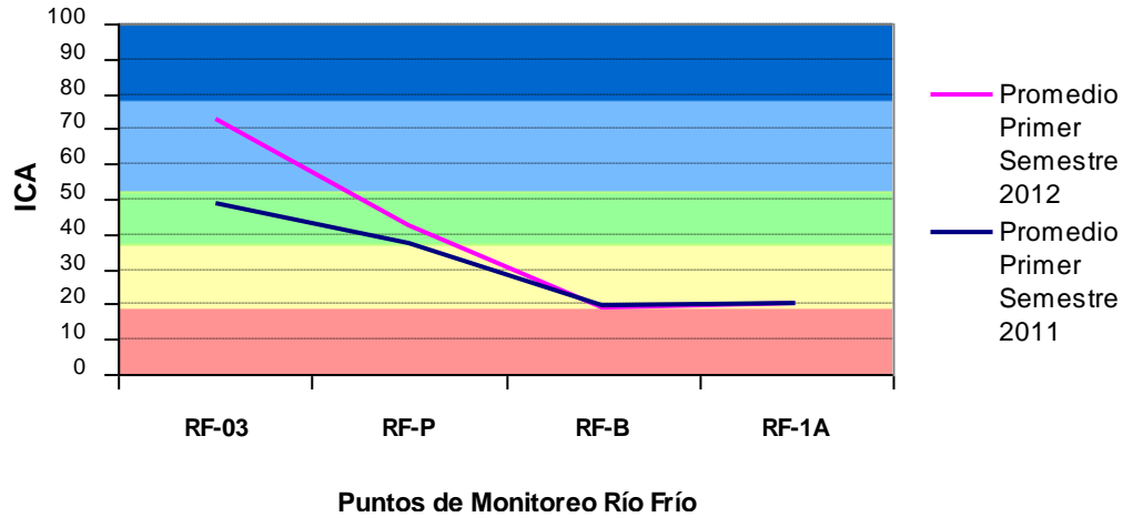
Gráfica 14. Índices de Contaminación del Agua Primer Semestre 2012- Río Frío
