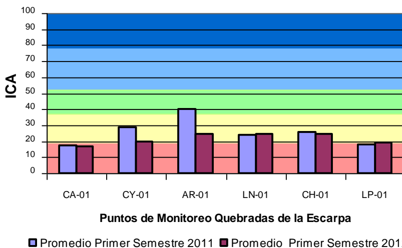
Gráfica 20. Promedio Índices de Contaminación del Agua - Quebradas de la escarpa
