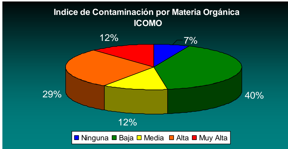
Gráfica 3. Promedio Índice de Contaminación por Materia Orgánica
