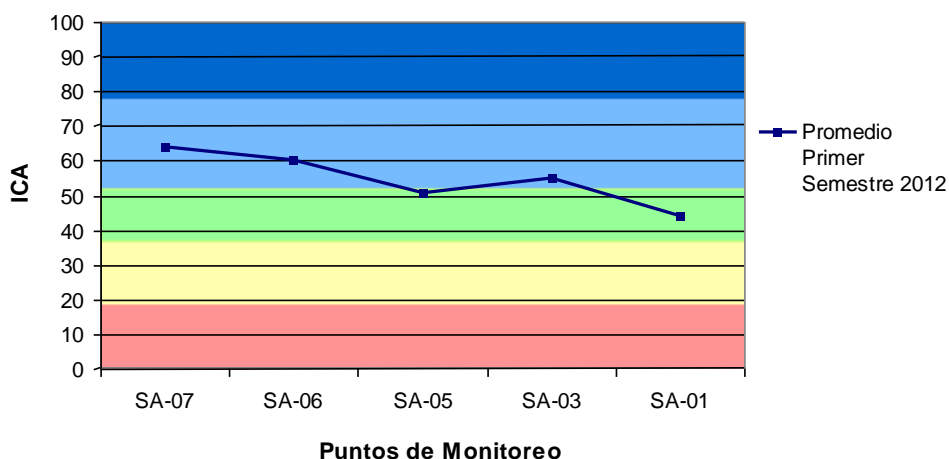
Gráfica 8. Promedio Índices de Contaminación del Agua - Río Suratá
