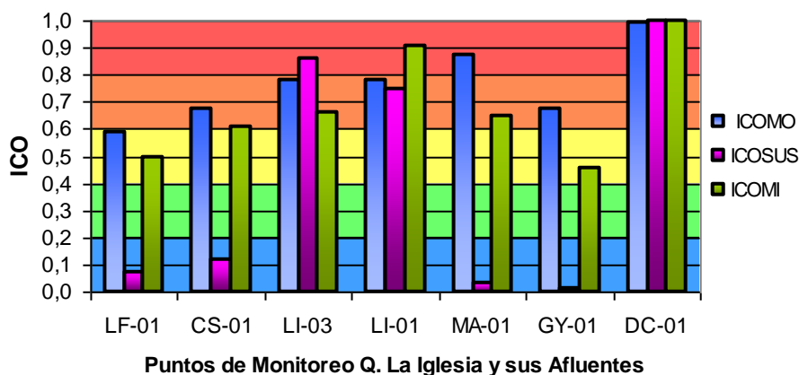
Gráfica 18. Promedio Índices de Contaminación del Agua - Qda La Iglesia y sus afluentes
