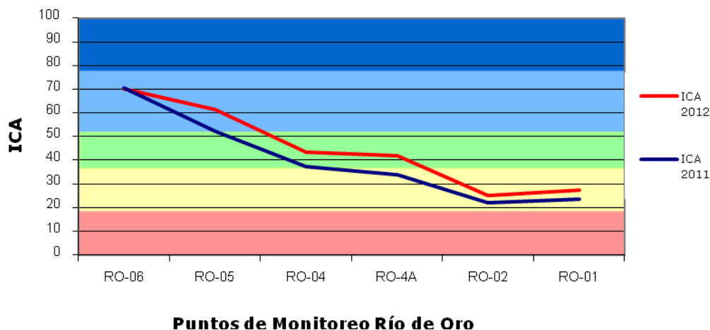
Gráfica 9. Promedio Anual Índice de Calidad del Agua - Río de Oro
