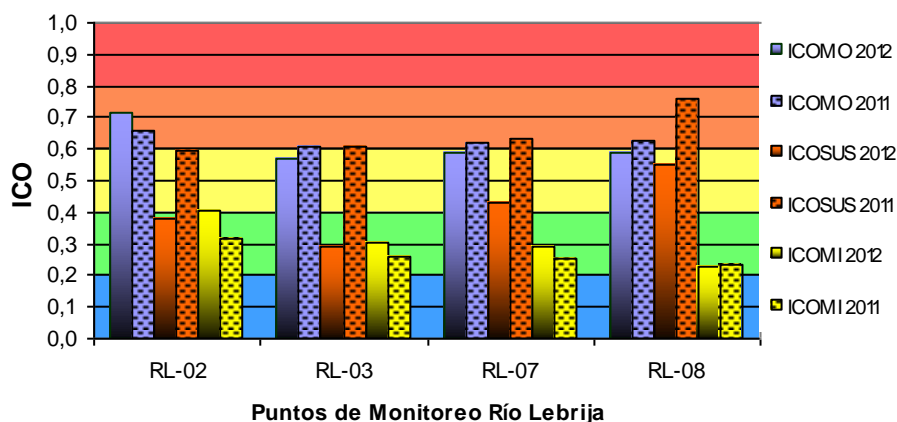
Gráfica 22. Promedio Índices de Contaminación del Agua 2012- Río Lebrija
