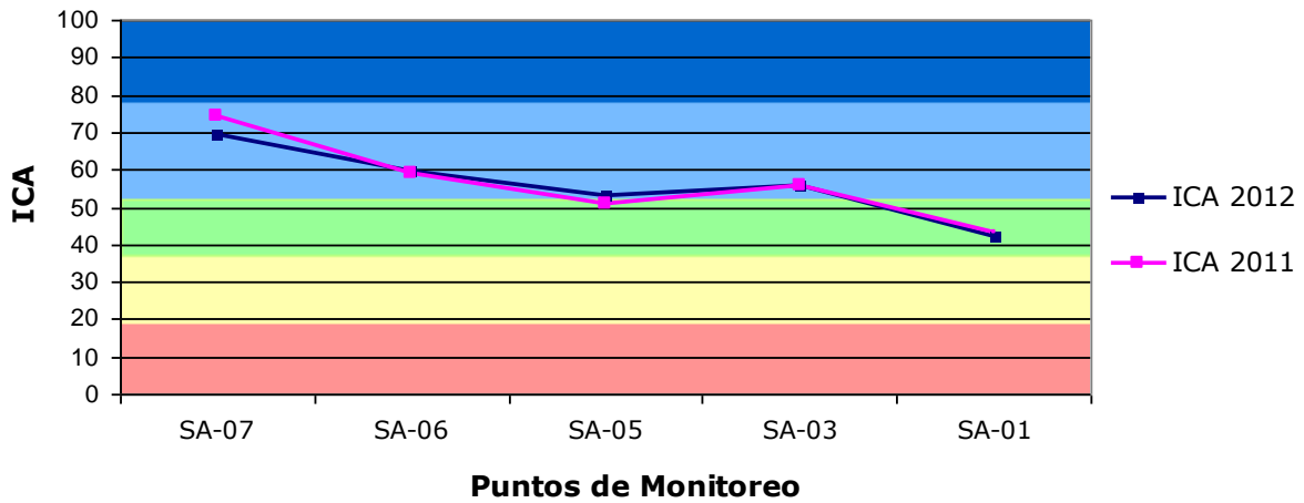
Gráfica 8. Promedio Índices de Contaminación del Agua - Río Suratá
