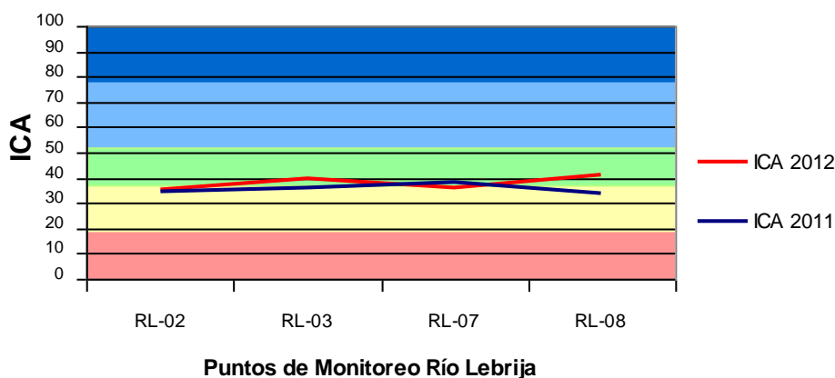
Gráfica 22. Promedio Índices de Contaminación del Agua 2012- Río Lebrija
