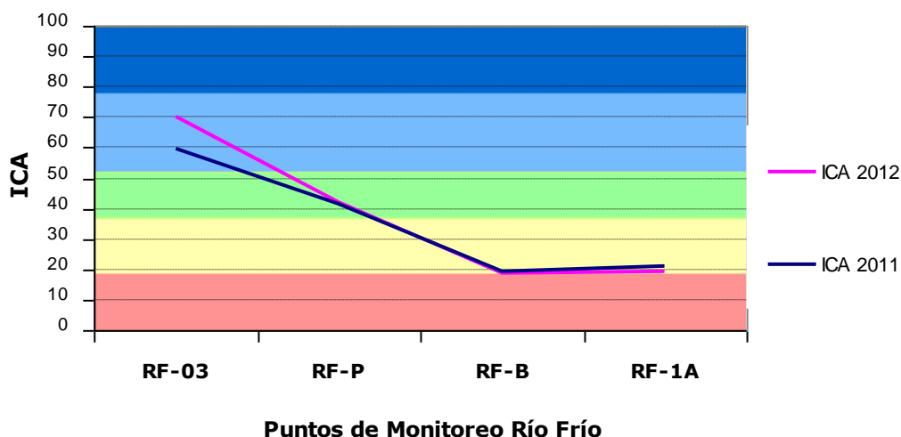
Gráfica 14. Promedio Índices de Contaminación del Agua 2012- Río Frío
