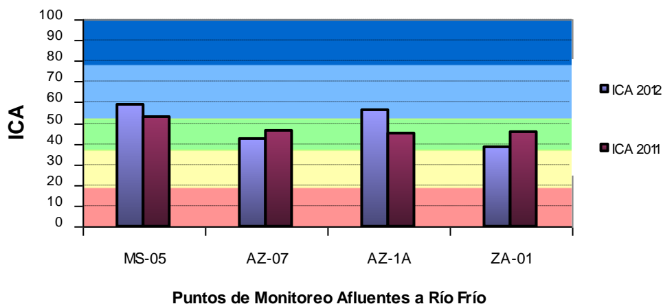
Gráfica 15. Promedio Anual Índice de Calidad del Agua – Afluentes Río Frío
