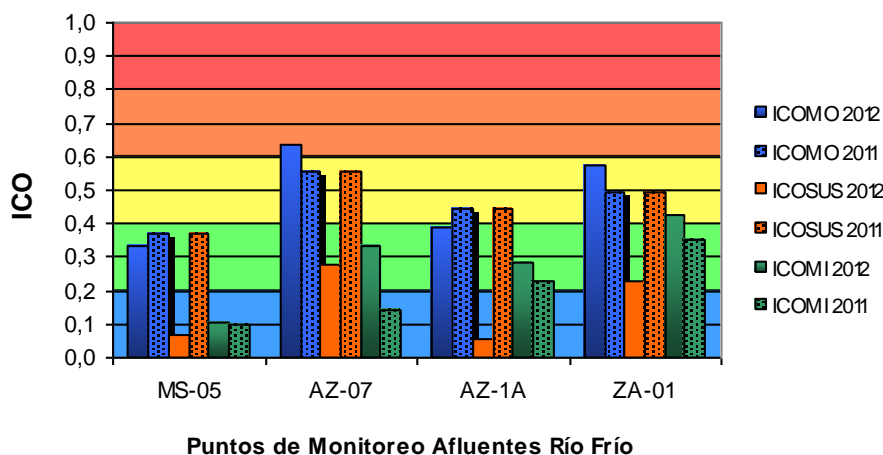
Gráfica 16. Promedio Índices de Contaminación del Agua 2012- Afluentes Río Frío
