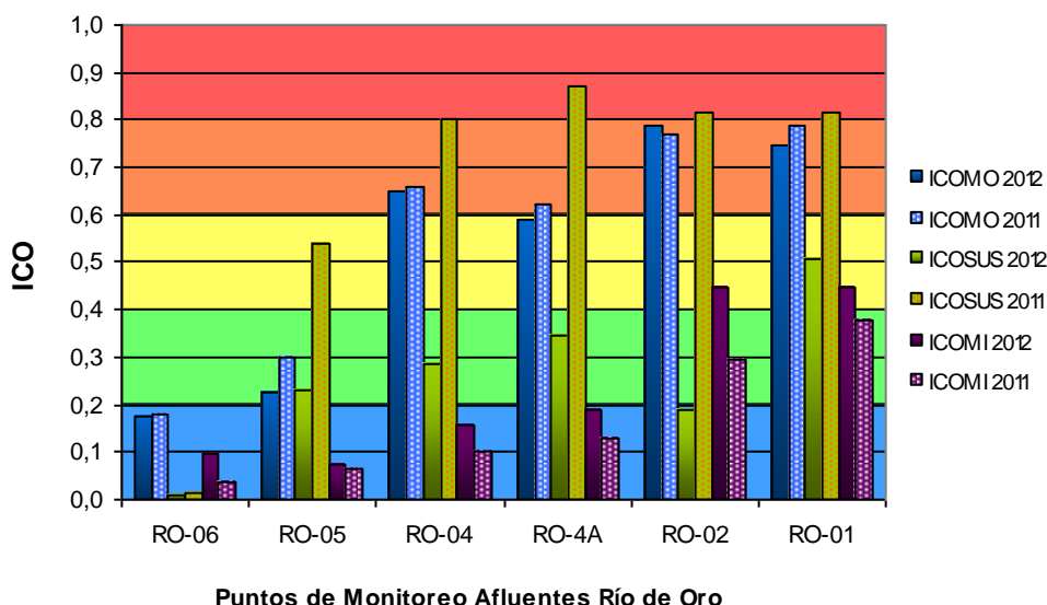
Gráfica 10. Promedio Índices de Contaminación del Agua - Río de Oro
